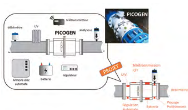
Schéma de principe solution Smart PICOGEN
